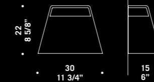
DIAPHANÈS A30 ED 13W 1300lm LED 2700K alimentatore dimmerabile dimmable ballast
