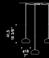
BOA S3D ED 3x9W 900lm LED 2700K CRI90 alimentatore dimmerabile dimmable ballast
