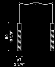
KIT DECENTRAMENTO DECENTRALIZATION KIT
