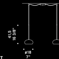
BOA S2D ED 2x9W 900lm LED 2700K CRI90 alimentatore dimmerabile dimmable ballast
